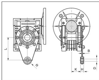
扭力臂 (A) 尺寸
