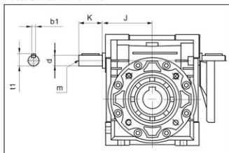
蜗轮输出轴 (DZ, SZ) 尺寸
